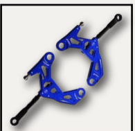
SAK-D6802/BU/V2 ALUMINIUM FRONT LOWER ARM FOR AUPER D6 BLUE AUPER D6 レッド用アルミフ ントロアーム (ブルー)
