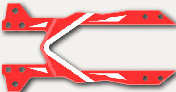
ALUMINIUM FRONT UPPER DECK [ 1 ] アルミフロントアッパーデッキ
