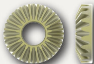
M0.6 X 20T 0.8-PITCH BEVEL GEAR [ 2 ] M0.6 X 20T 0.8ピッチベベルギア
