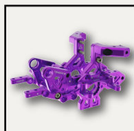
SAK-D6808/PU BELT DRIVE BULKHEAD FOR AUPER D6 PURPLE AUPER D6 用ベルトドライ バルクヘッド (パープル)
